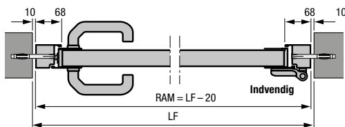
Separat dør med aluminium-standardkarm profiltype 2 Montering i åbningen
